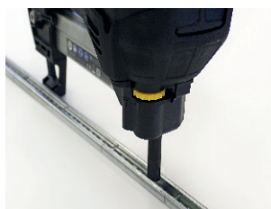
Regulator de adâncime de înaltă precizie
